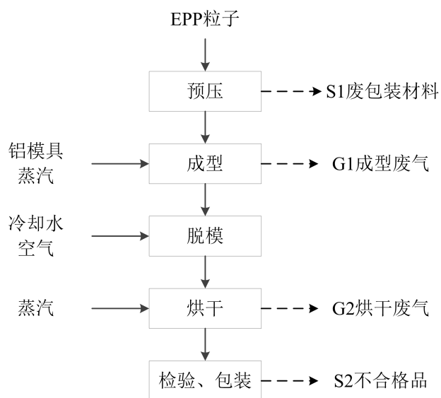
图 2-3 生产工艺流程及产污环节图（图注：G-废气，S-固废）
